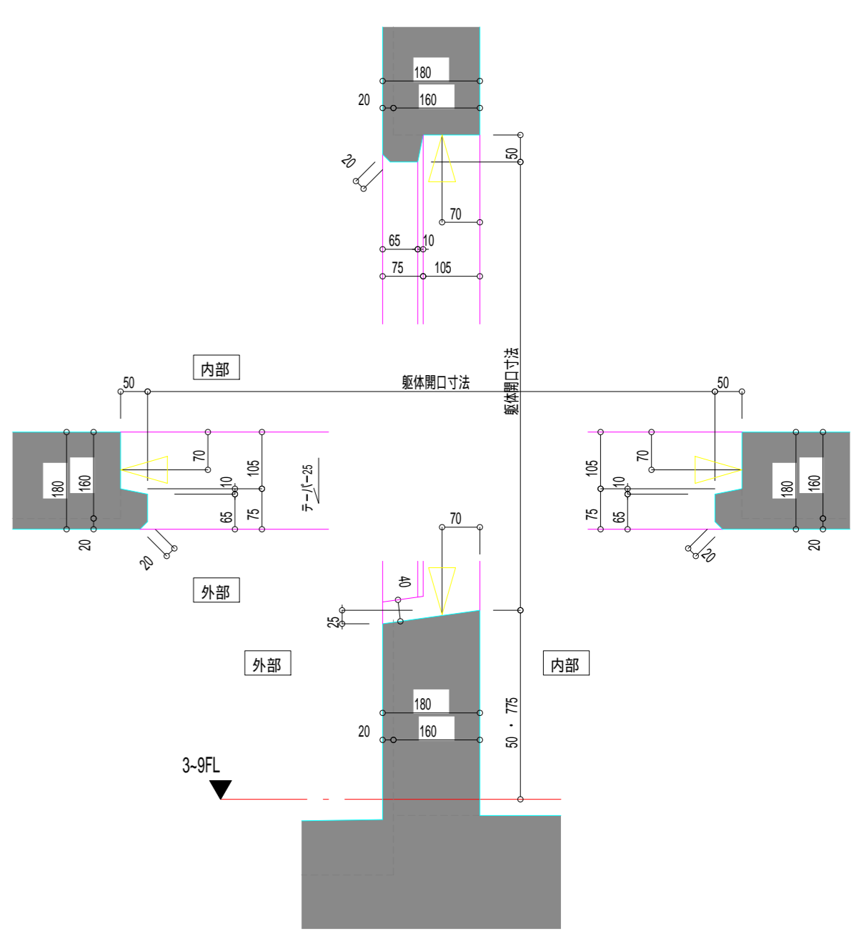
外壁開口部詳細図
