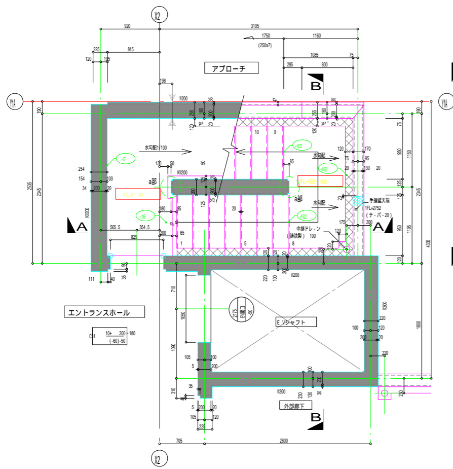
(屋外階段A) 1階床伏せ図 s=1/30
