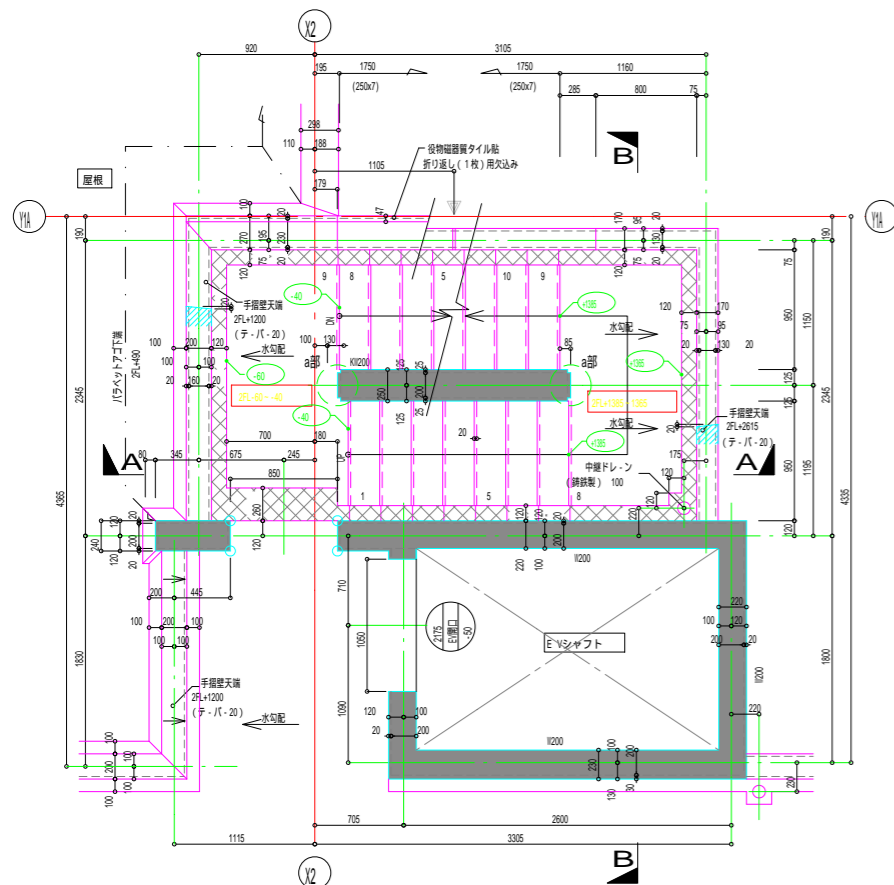
(屋外階段A) 2階床伏せ図 s=1/30
