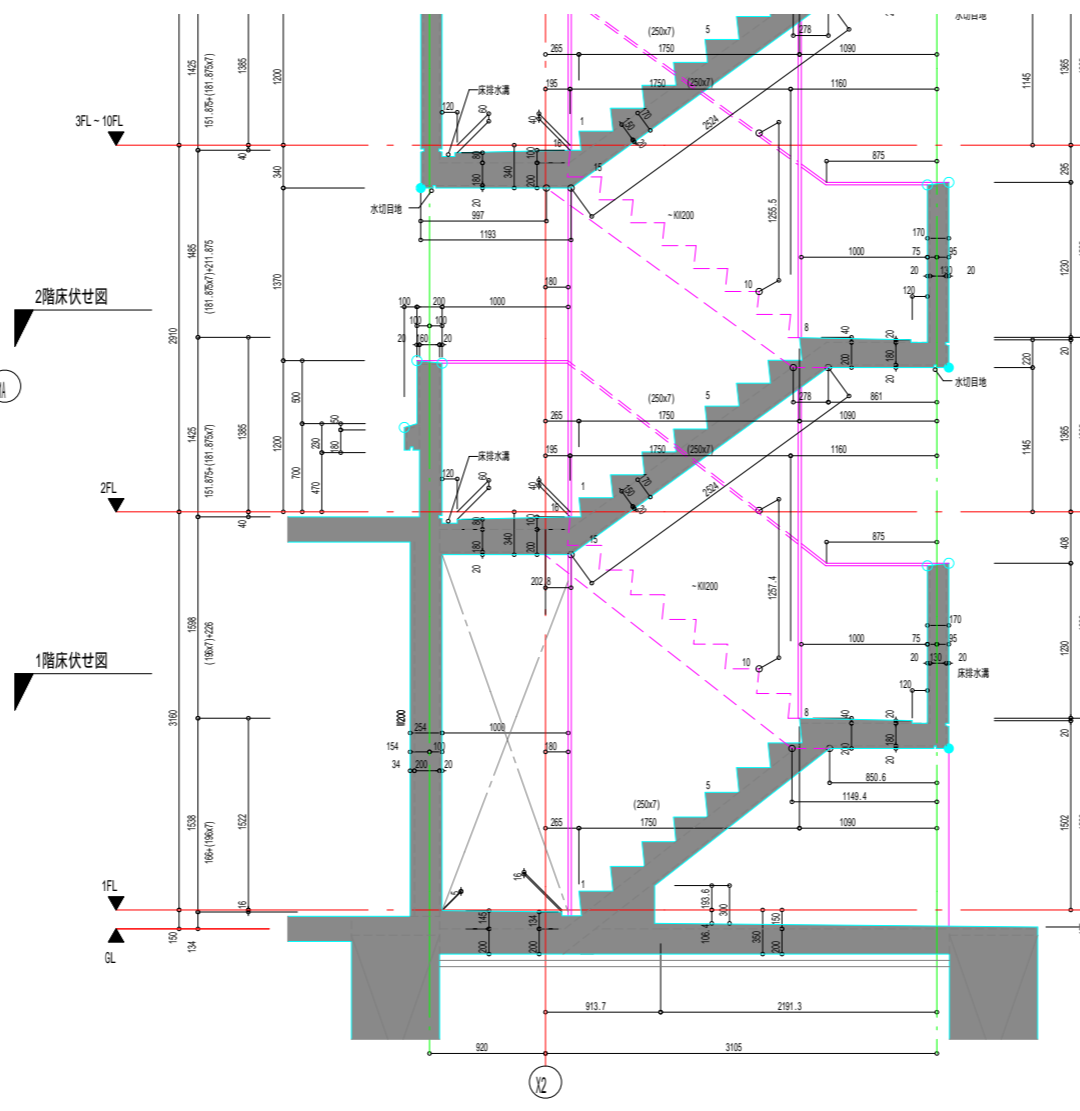
A-A 断面図 s=1/30
