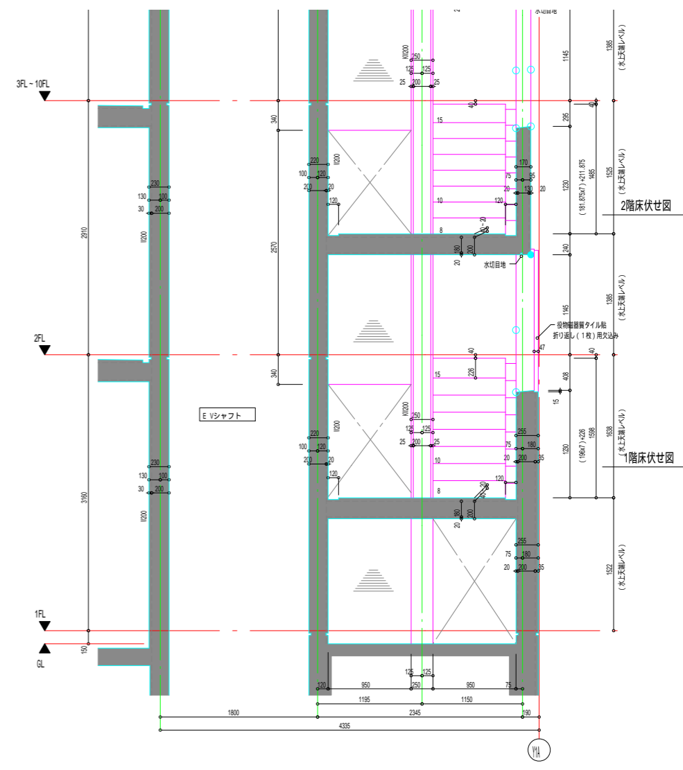
B-B 断面図 s=1/30
