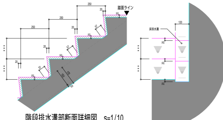
階段排水溝断面詳細図 s=1/10
