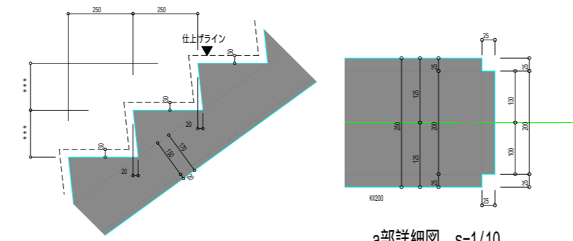
階段断面詳細図 s=1/10
